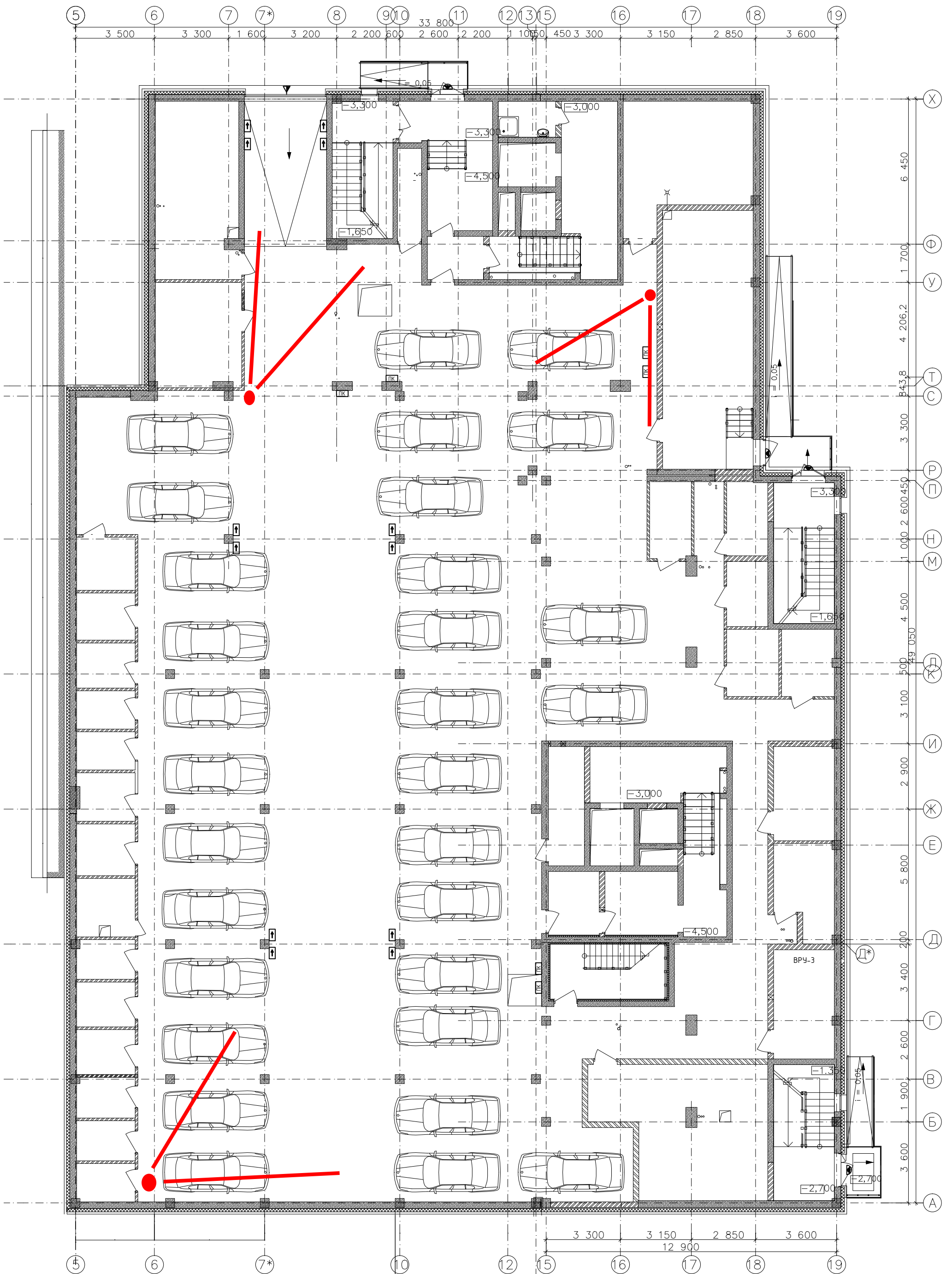
План этажа на отм. -4,500
